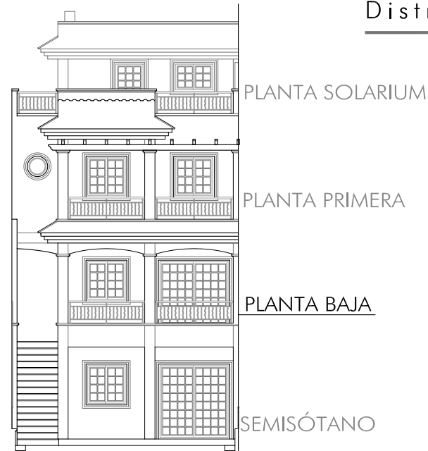
ALZADO DE LA VIVIENDA VILLA
